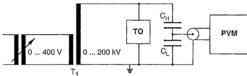
Фиг. 4.2.: Схема на свързване за изпитване при променливотоково напрежение T_1 : трансформатор 400V/200 000V; 60 kVA; u_K=3,5 \% ; 50 Hz C_H : 180 pF; съотношение 2000:1; PVM: Амплитуден волтметър TO: Тестван обект, отклонение при измерване около 3%
