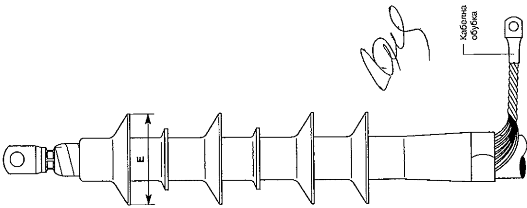
3M PST QT II Тяло на кабелната глава
