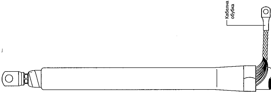
3M PST QT II Тяло на кабелната глава
